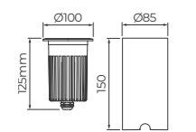
Dimensão do corte: Ø76mm (3")
