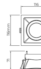
Dimensão do corte: 100x100mm
