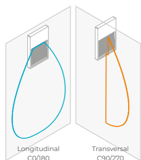
Ilustração 3 – Neu 2 | Balizador de Sobrepor STH8750/30
