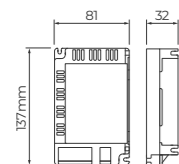
Diagrama de instalação
