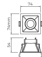
Dimensão do corte: 62x62mm
