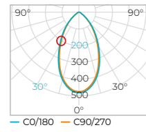
Gráfico 2 – Dicroica MR16 ECO STH8538/30
