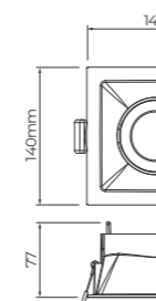
Dimensão do corte: 127x127mm
