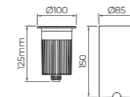
Dimensão do corte: Ø76mm (3")
