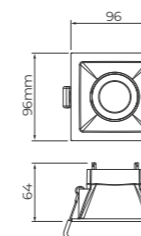
Dimensão do corte: 80x80mm
