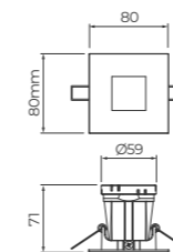
Dimensão do corte: Ø64mm (2.1/2")
