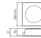
Dimensão do corte min.: Ø50,8mm (2")
