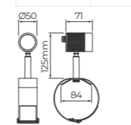
Diâmetro máximo da cinta: Ø130mm
