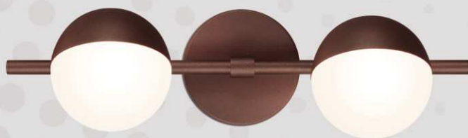
ARANDELA PALANI 1462 Porta lâmpadas: 2 x G9 Halopin Difusores: Globos de vidro branco opalino Ø 100 mm Luminária total: ⇄ 100 x ↔ 400 mm Base de parede: Ø 100 x 15 mm Profundidade: ↗ 145 mm
